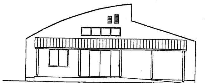
北立面図
